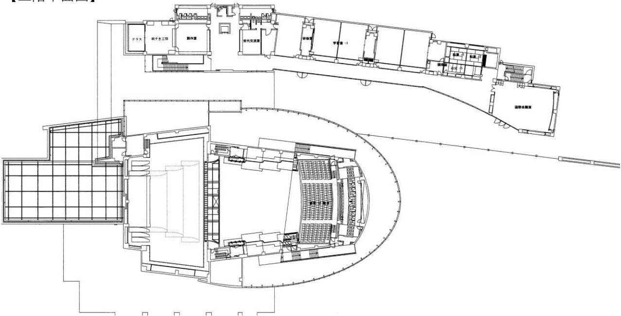
【三階平面図】
